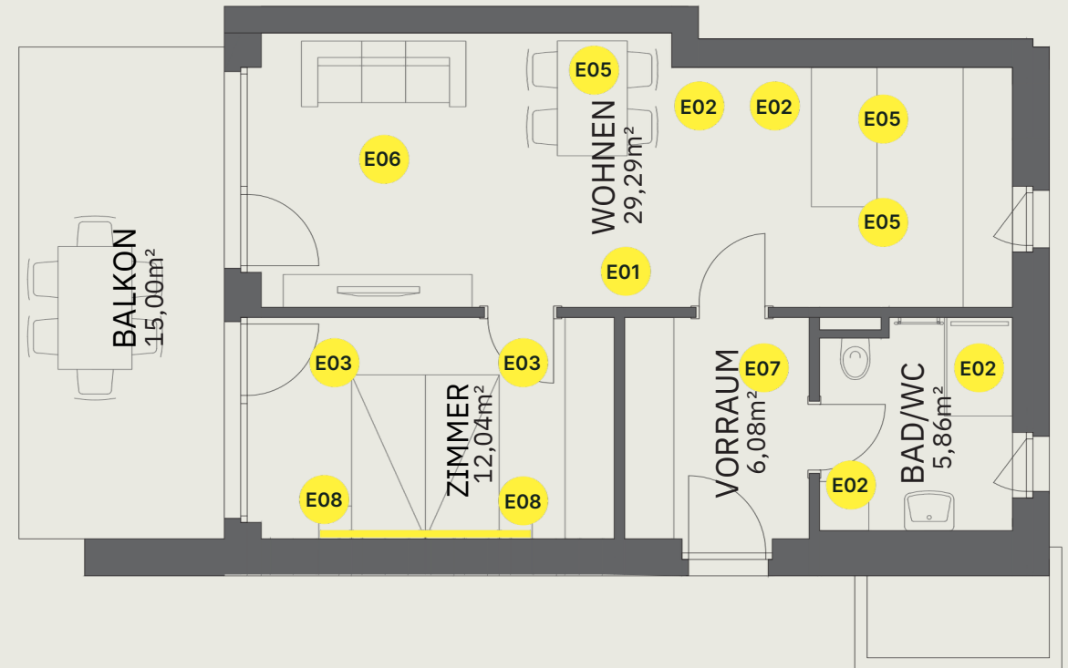
Beispiel - Top 05: 2D Lichtplanung
